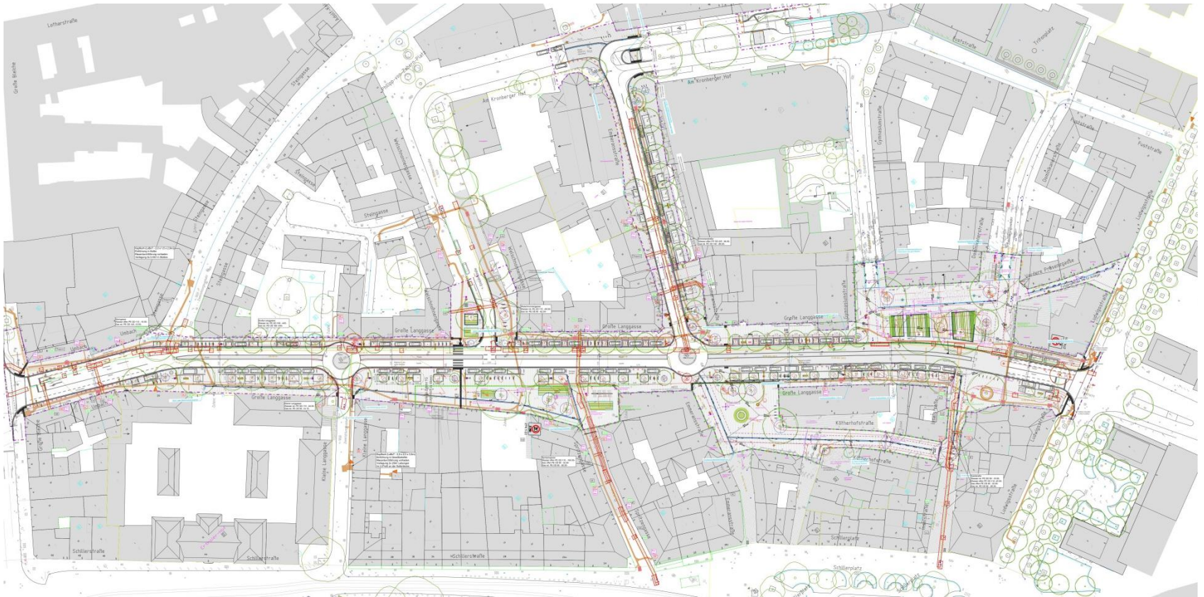
Leitungsplan
