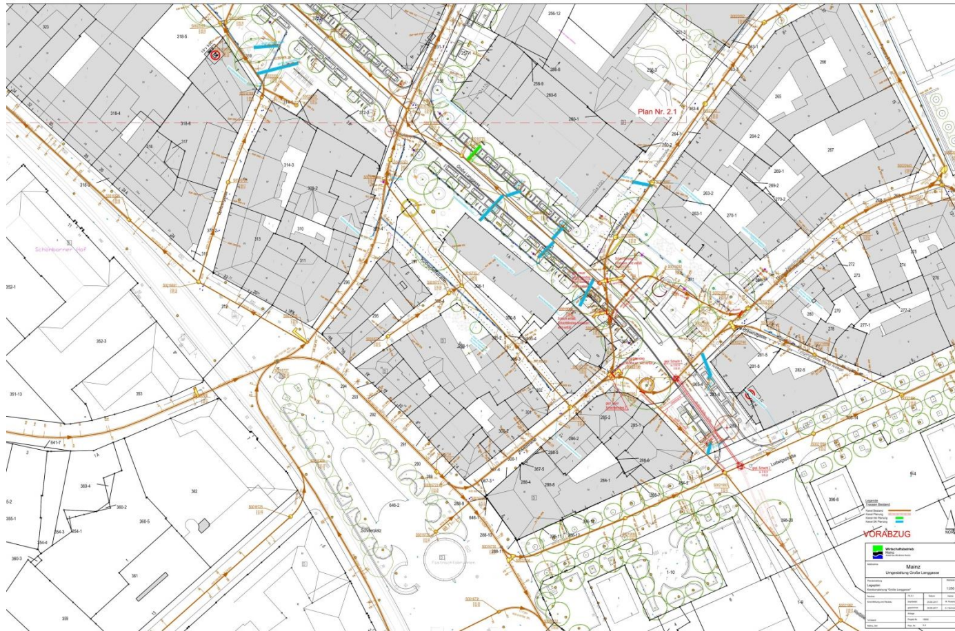
Kanalplan Süd
