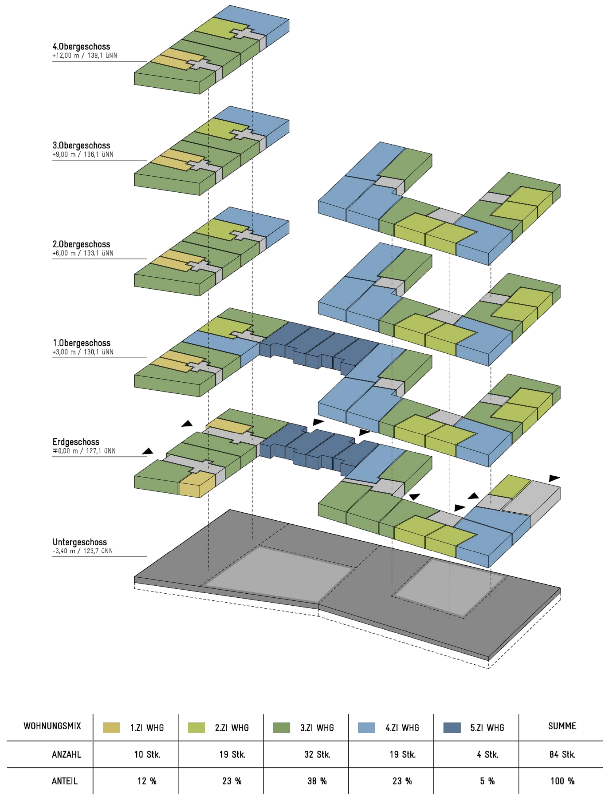
Isometrie Wohnungsmix
