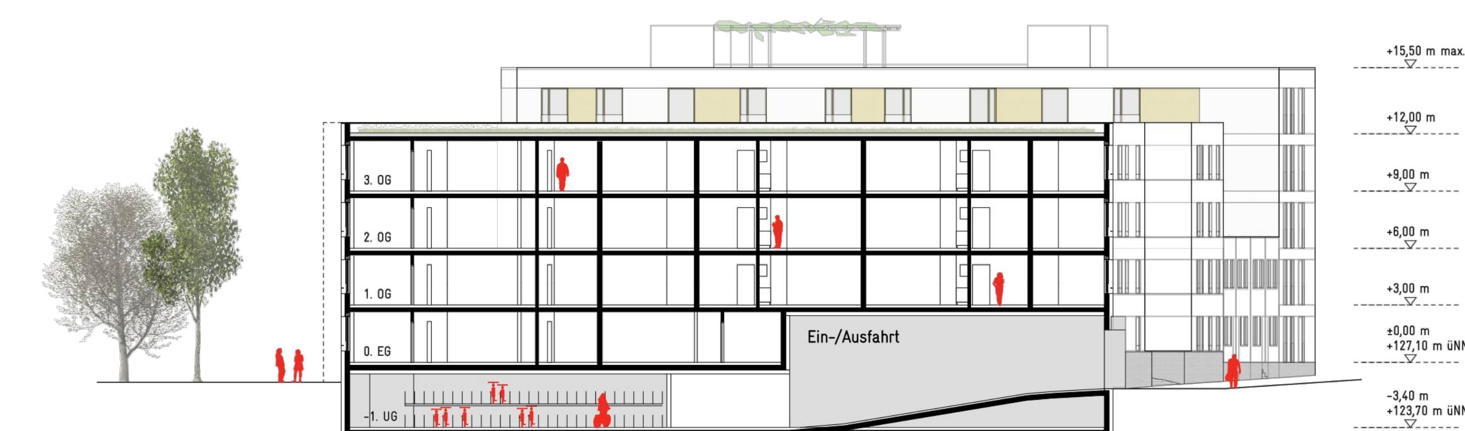
B-B Schnitt | M.1:200
